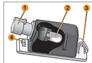
Рис. 17. Фонарь освещения номерного знака
