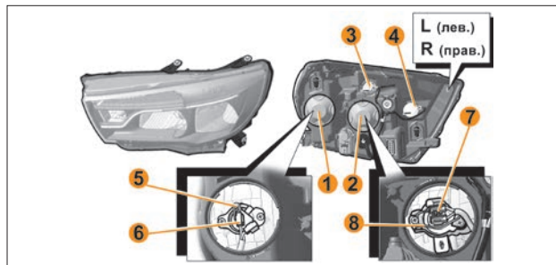
Рис. 11. Блок-фара
